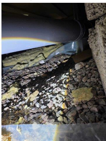
Bild 5: - Utvändigt, Grundmur/Hussockel, Krypgrund, se riskanalys Fuktmärken på trossbotten vänster om inspektionslucka. Markplats saknas ...
