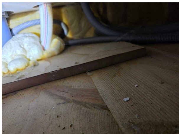
Bild 21: - Invändigt, Entréplan, Läckage på vattenslang till diskmaskin. (Torrt vid besiktningstillfället) Otäta rörgenomföringar ...
