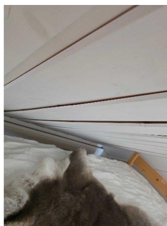
Bild 24: Invändigt, Loft, Innertak dåligt spikat.
