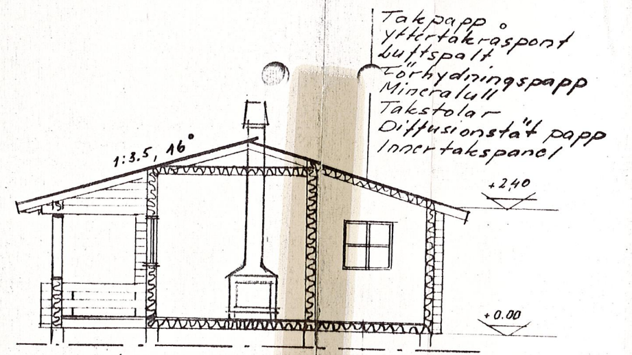
Sektion A-A
